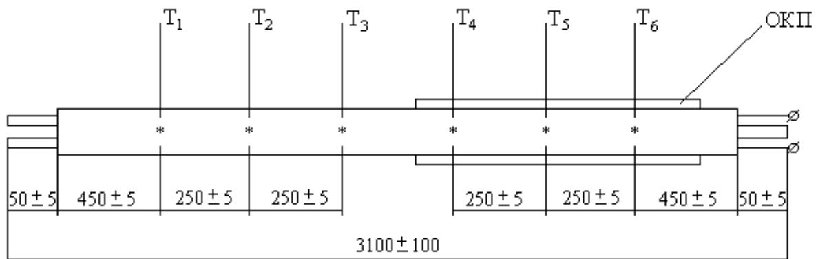
Размещение термоэлектрических преобразователей
